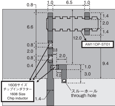
電極パターン(基板表面): AM11DP-ST01*[特許取得済み] Land pattern (Surface of the Substrate) [Patented]
