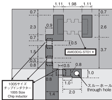
電極パターン(基板表面): AM03DP-ST01*[特許取得済み] Land pattern (Surface of the Substrate) [Patented]
