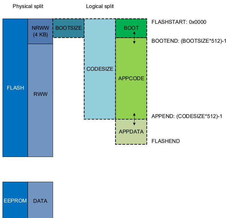
Figure 11-2. AVR DU Flash Memory Map
