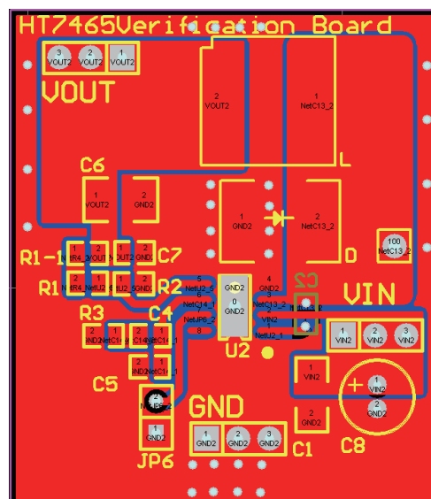
Top Layer
