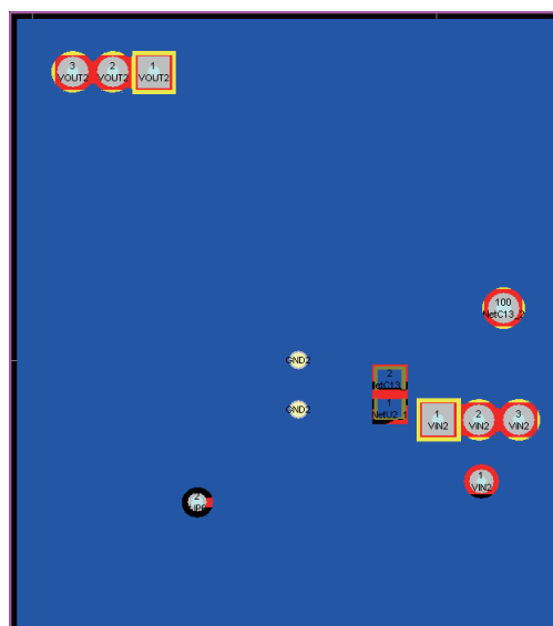
Bottom Layer
